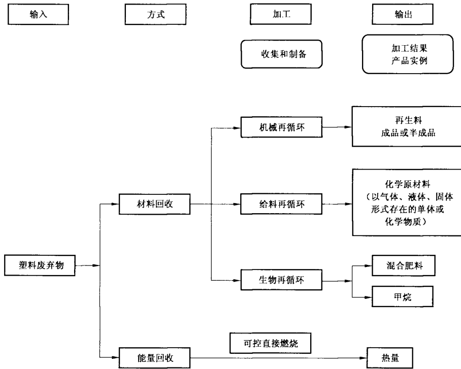
图 A.1 一些塑料回收方式的示意图
